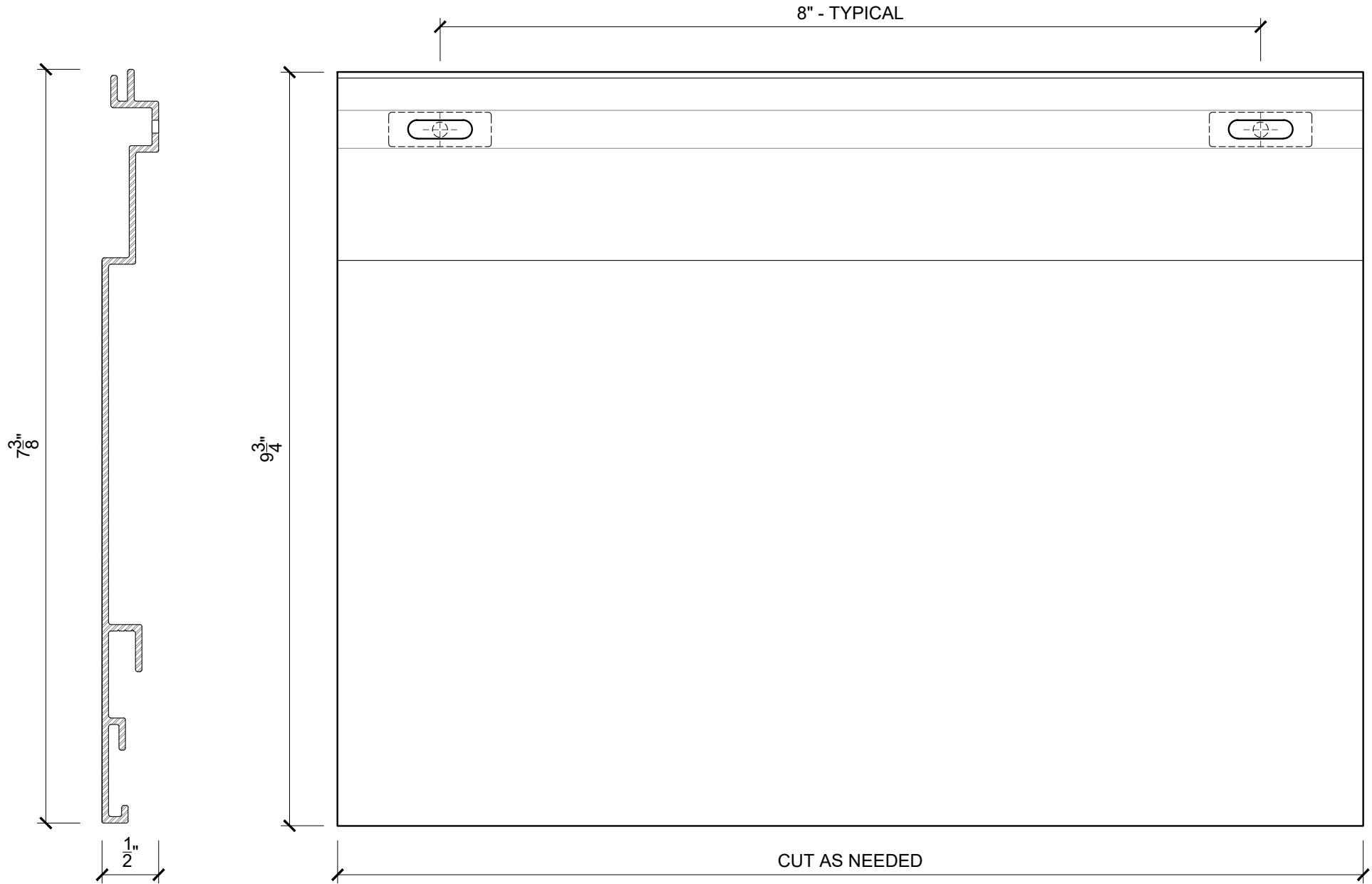
1 PL1 - PROFILE PL1-A SCALE 9"=1'-0"
